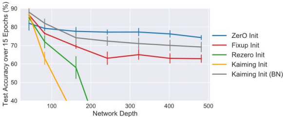
Обучение ultra deep ResNet на CIFAR-10 15 эпох
